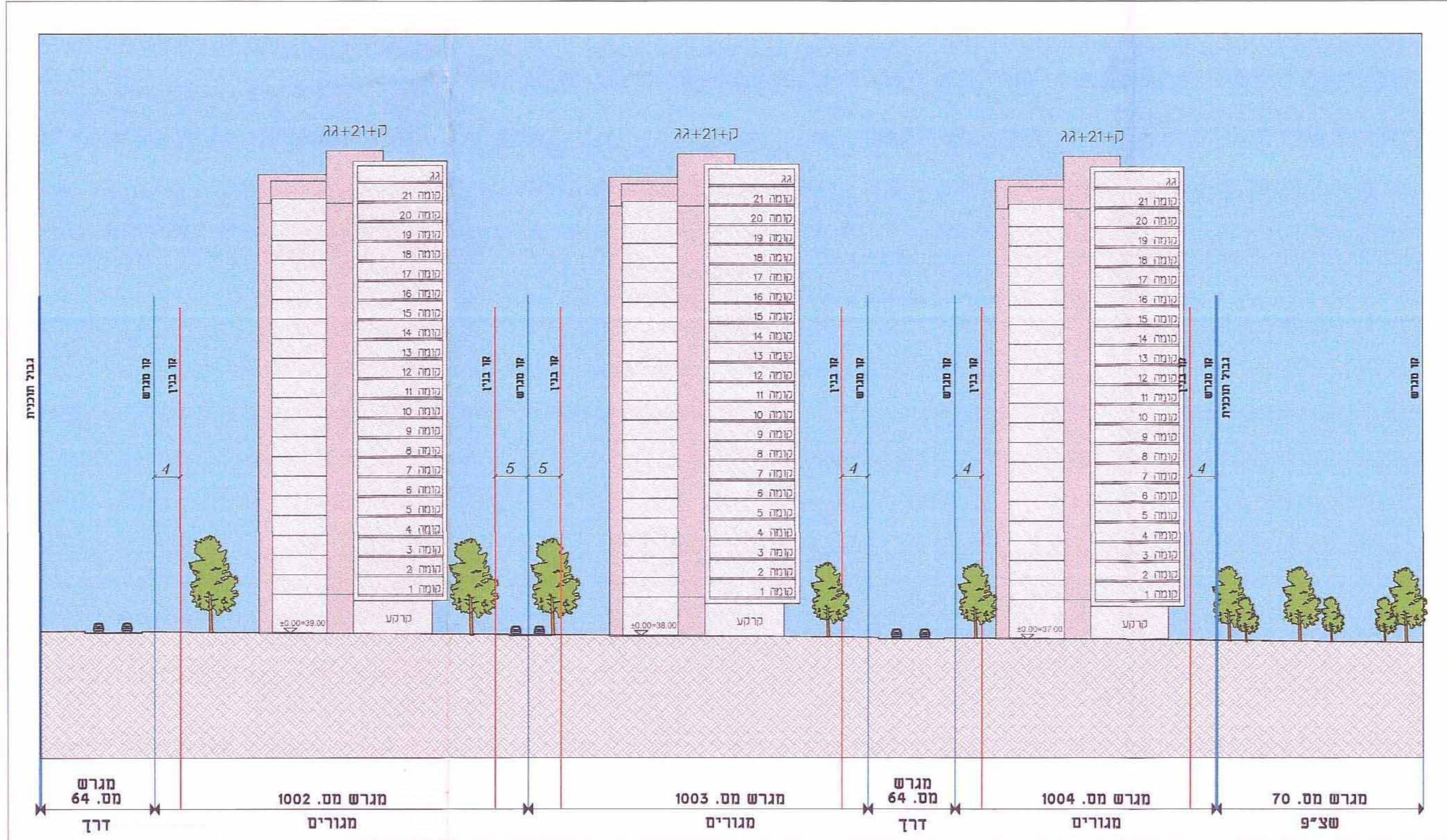
חתך 1-1, קנ"מ 1:500
