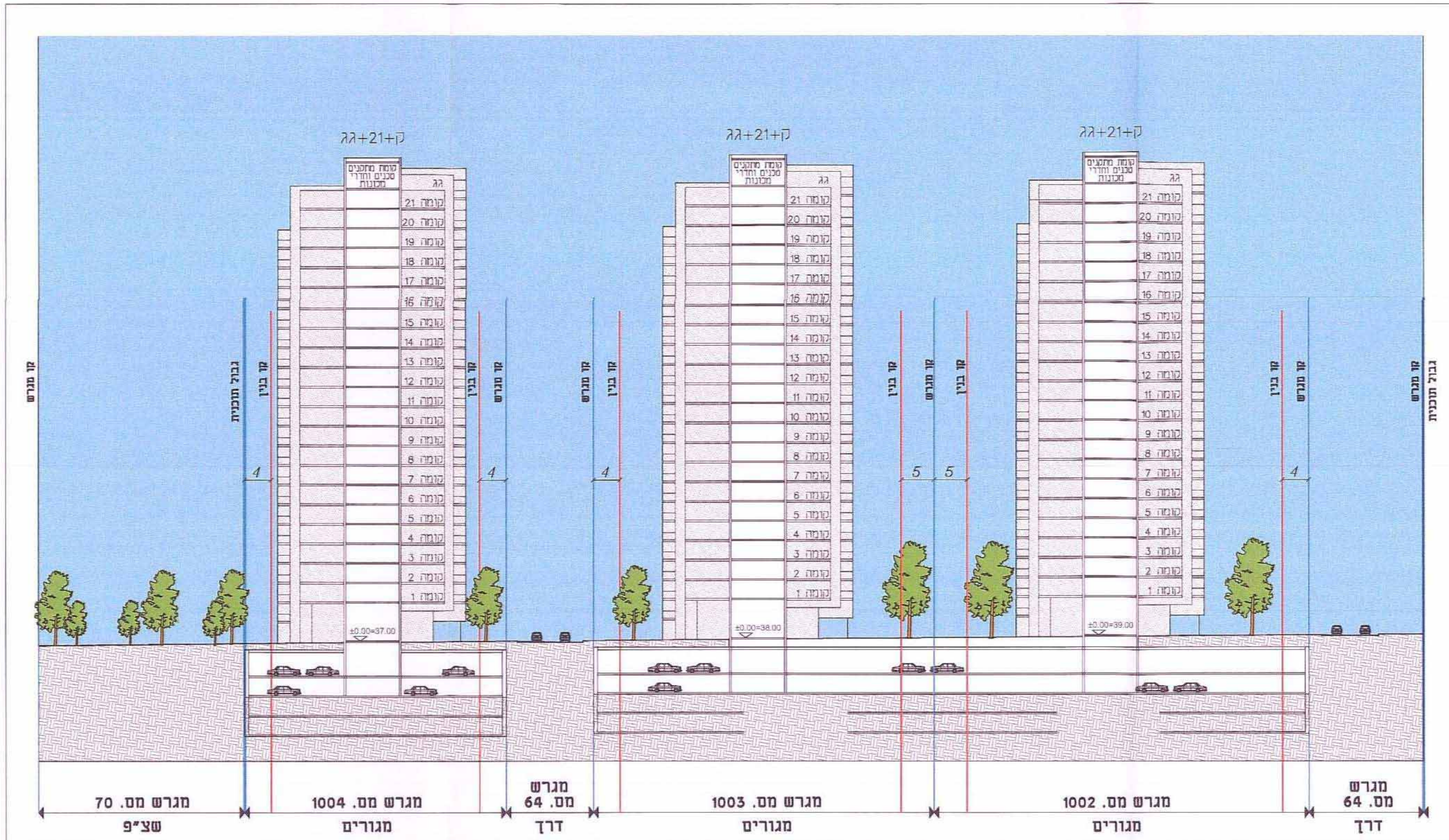
חתך 2-2, קנ"מ 1:500
