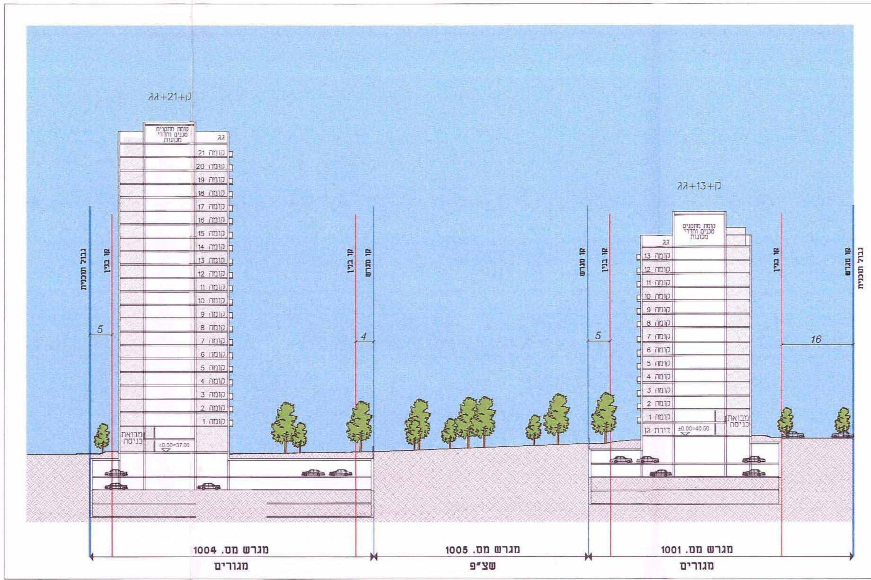
חתך 4-4, קנ"מ 1:500
